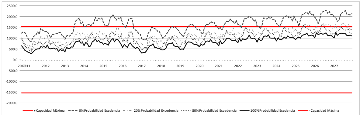
Figura 7: Flujos con probabilidad de excedencia Transformador 500/220 subestación Alto Jahuel, Periodo 2010-2027.
