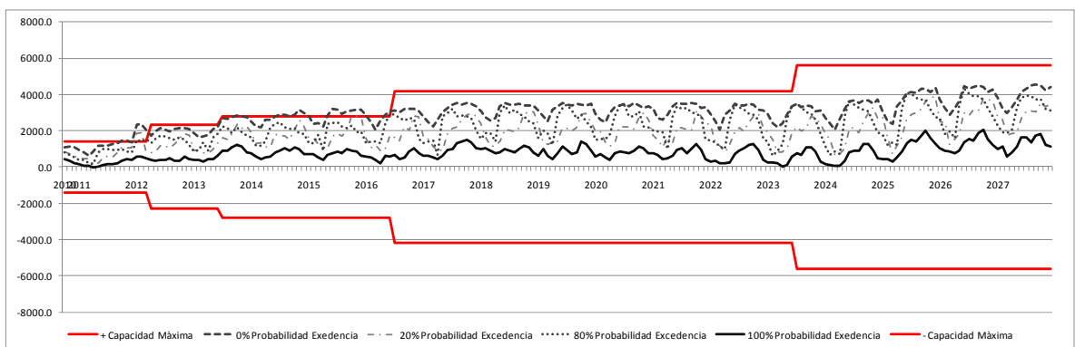
Figura 5: Flujos con probabilidad de excedencia línea Ancoa-Alto Jahuel, Periodo 2010-2027.
