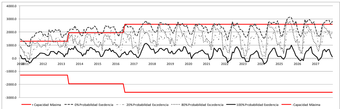
Figura 9: Flujos con probabilidad de excedencia Transformador 500/220, subestación Charrúa, Periodo 2010-2027
