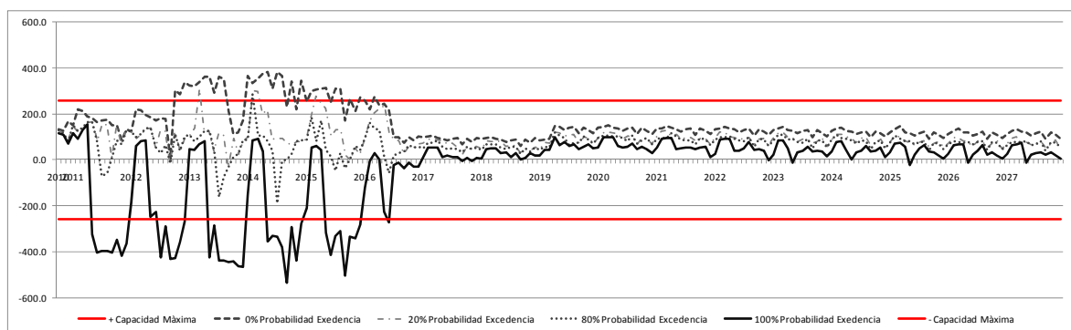
Figura 2: Flujos con probabilidad de excedencia línea Maitencillo-Punta Colorada, Periodo 2010-2027.
