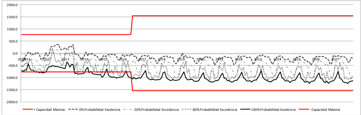
Figura 8: Flujos con probabilidad de excedencia Transformador 500/220 subestación Ancoa, Periodo 2010-2027.
