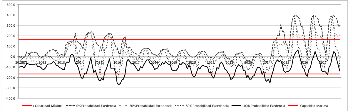
Figura 10: Flujos con probabilidad de excedencia línea Ciruelos-Cautín, Periodo 2010-2027.
