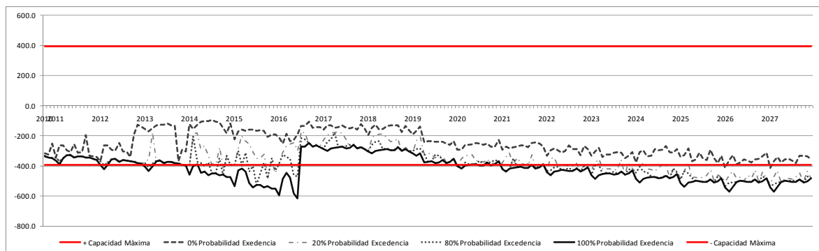
Figura 1: Flujos con probabilidad de excedencia línea Cardones-Maitencillo, Periodo 2010-2027
