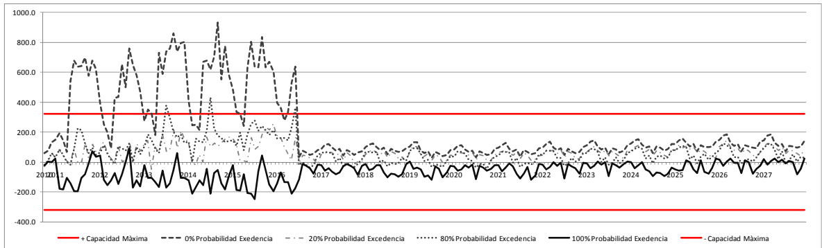
Figura 4: Flujos con probabilidad de excedencia línea Nogales-Los Vilos, Periodo 2010-2027.
